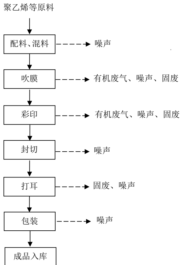
图 2-2 塑料袋生产工艺流程及产污环节图
