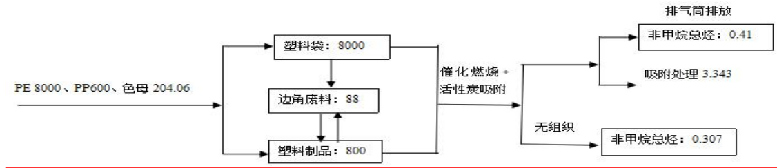
图 2-2 项目物料平衡图 单位: 吨/年
