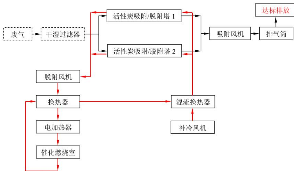
图五 催化燃烧设备工艺流程图
