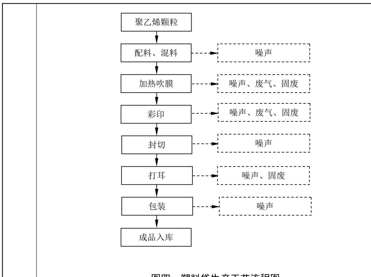
图四 塑料袋生产工艺流程图
