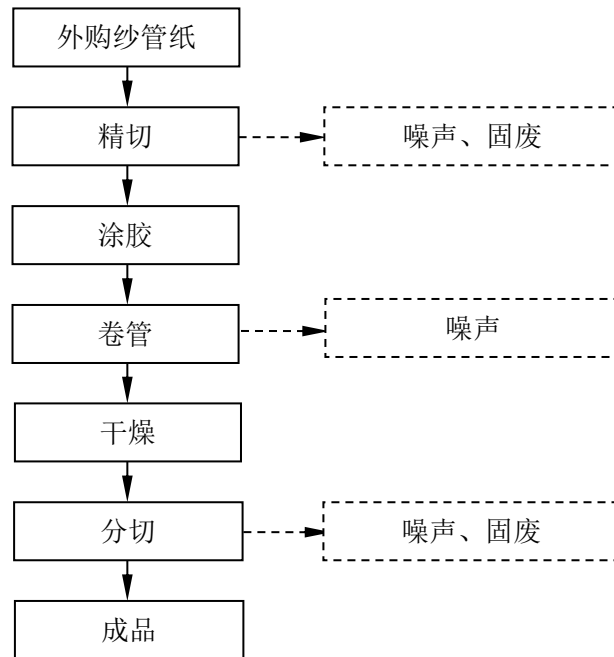
图五 纸管生产工艺流程图
