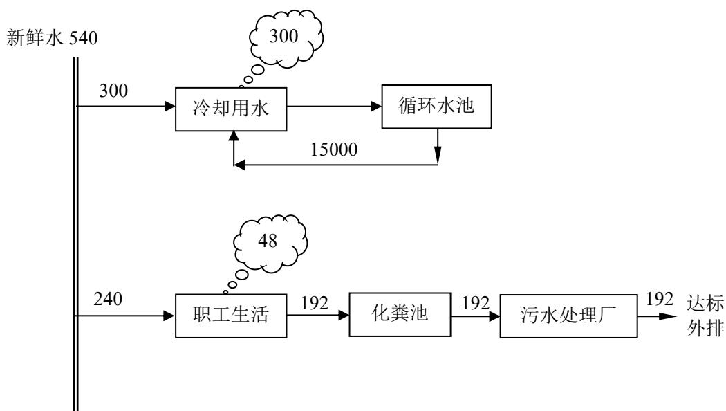
图一 本项目水平衡图 (单位: m 3 /a; ☁ 表示蒸发损失量)
