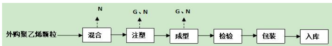
图 2-5 塑料制品生产工艺及产污流程图
