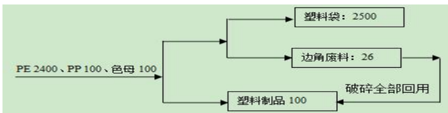
图 2-2 项目物料平衡图 单位：吨/a
