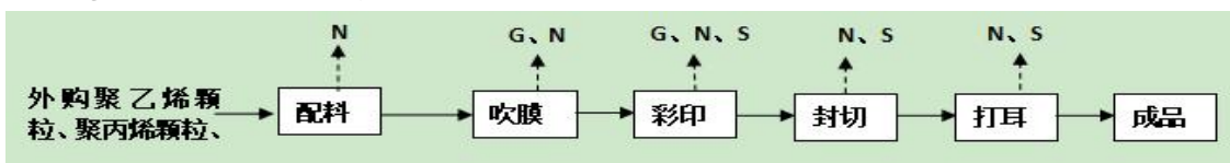
图 2-3 塑料袋生产工艺及产污流程图
